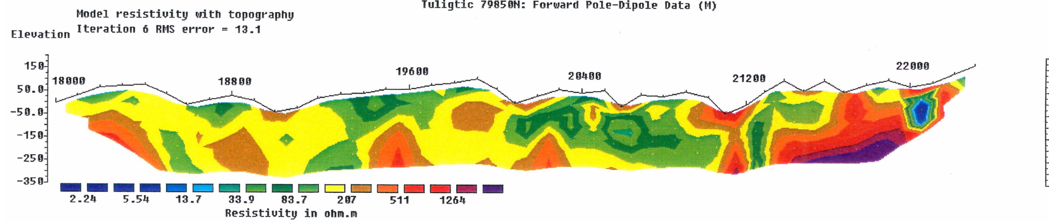
Tuligtic 79850N: Forward Pole-Dipole Data (M)
